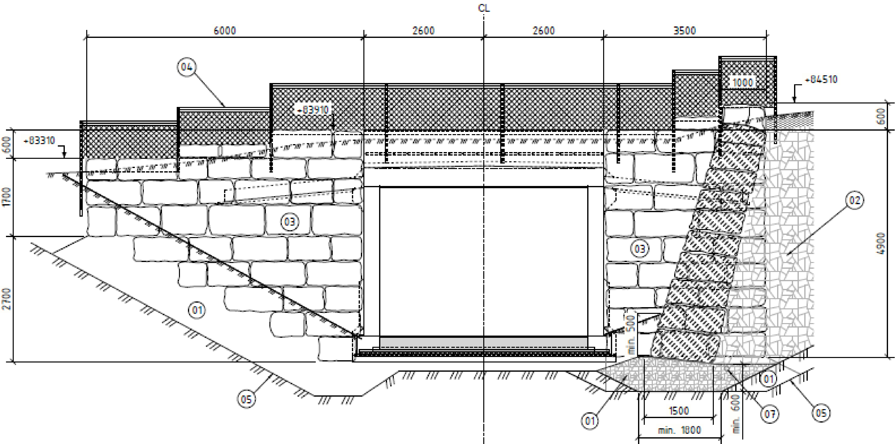
SNITT A - A 150
