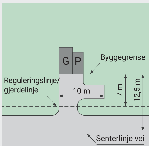
Hovedprinsipp for plassering av garasje, biloppstillingsplass og snuplass på egen grunn.
