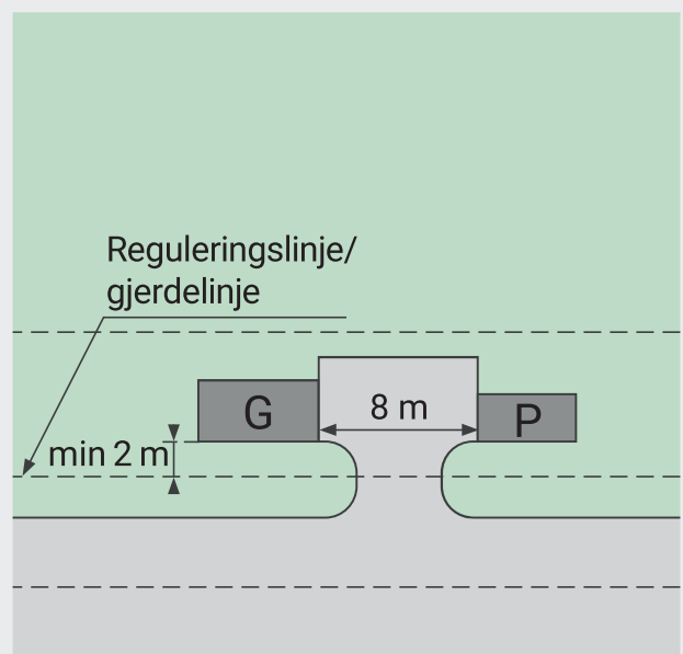
Hovedprinsipp for plassering av garasje, biloppstillingsplass og snuplass på egen grunn.
